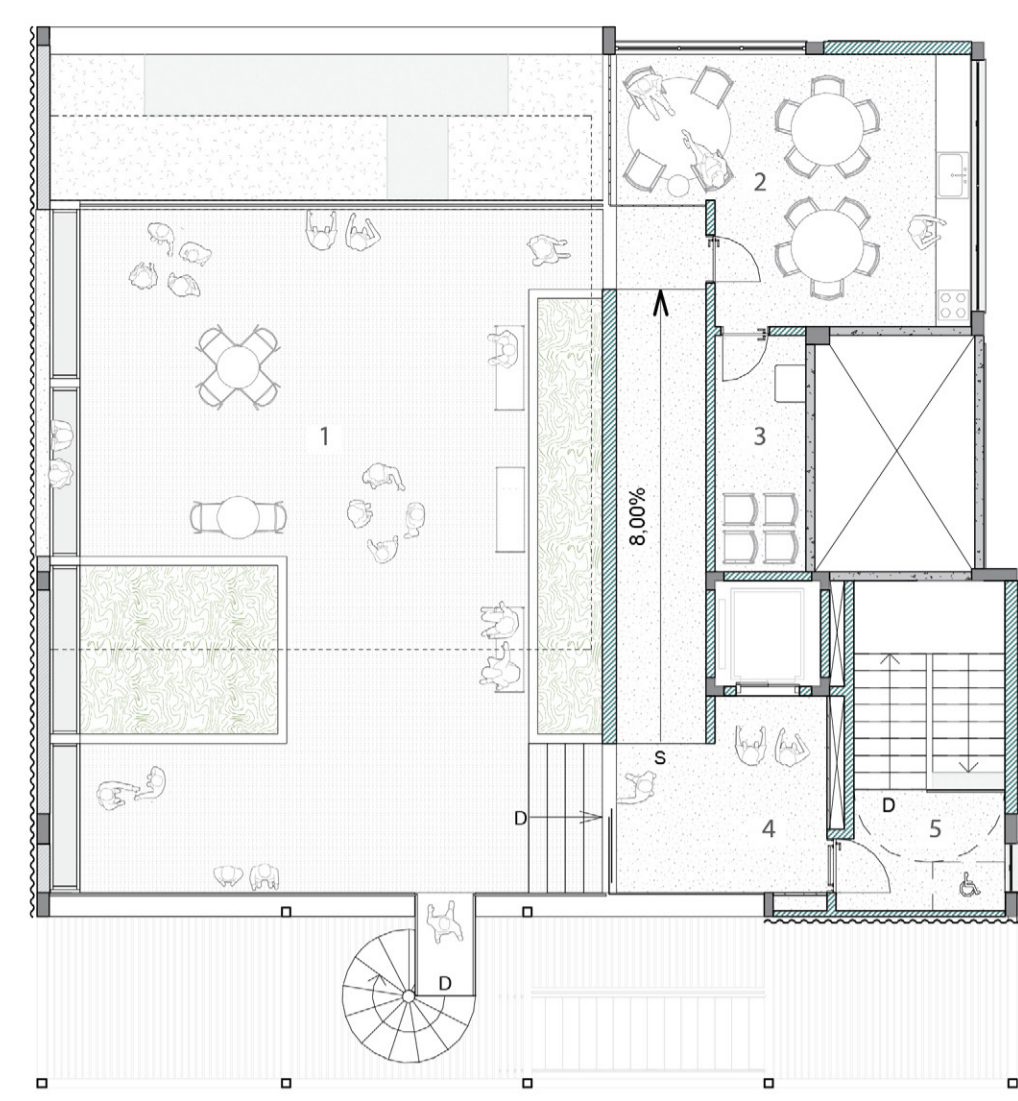
PLANTA TERRAÇO . 1/125
