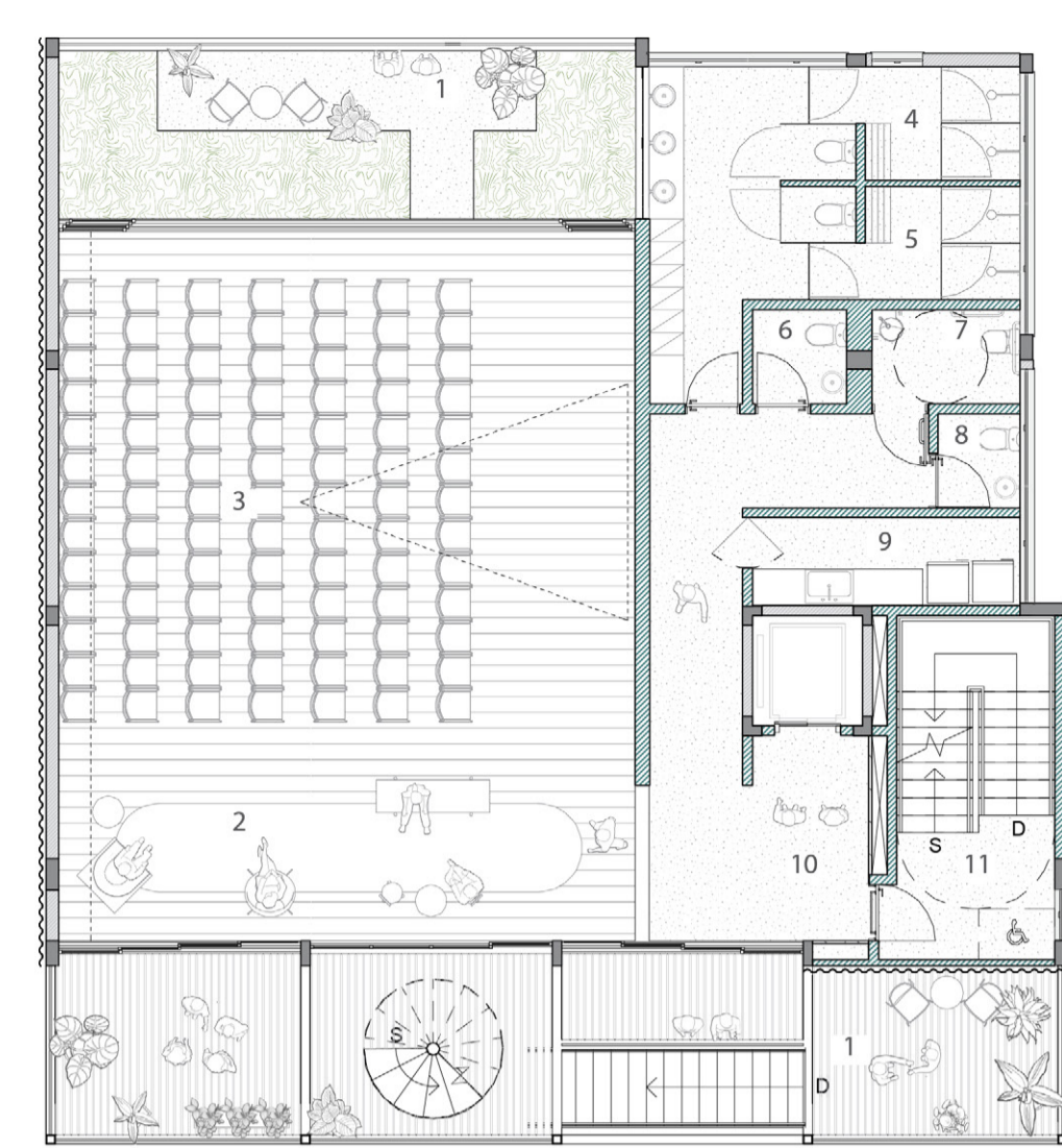
PLANTA 5º PAVIMENTO . 1/125
