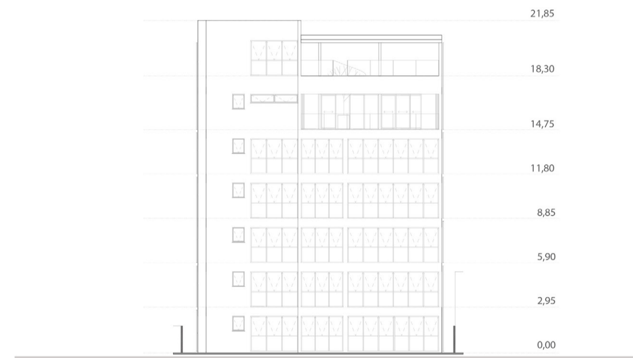
FACHADA SUL . 1/250
